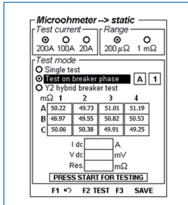
Microhmmeter display
